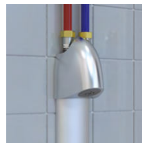
Aufputz-Wasseranschlüsse
