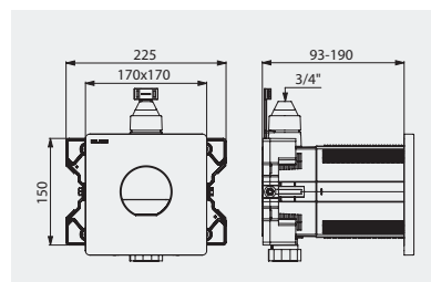
TEMPOFLUX 3 für Unterputzmontage Metall verchromt Art. DELABIE: 763BOX-763040
