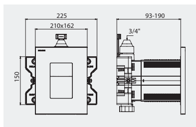
TEMPOFLUX 3 für Unterputzmontage Edelstahl satiniert Art. DELABIE: 763BOX-763000
