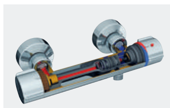
Querschnitt H9769: geringes Wasservolumen, thermische Isolierung und keine Rückflussverhinderer erforderlich Art. DELABIE: Coupe3D_H9769
